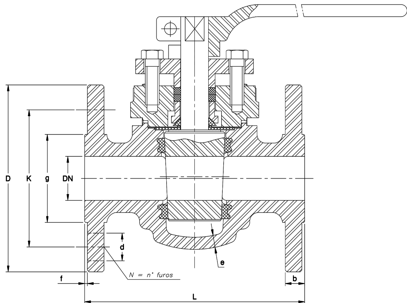
Válvula Macho 150 lbs/pol²
