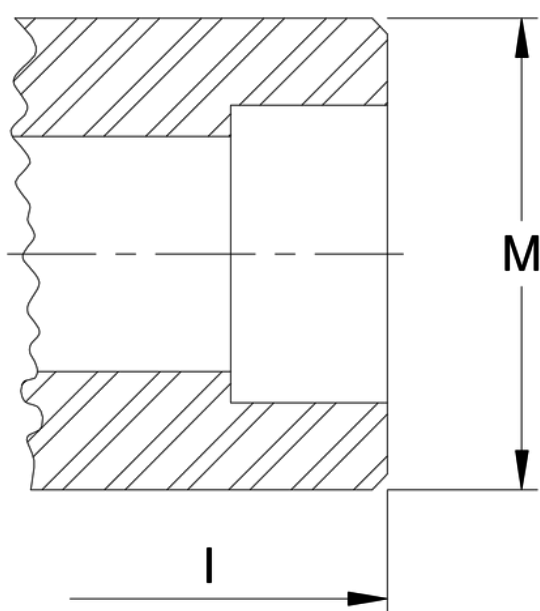
ENCAIXE PARA SOLDA
